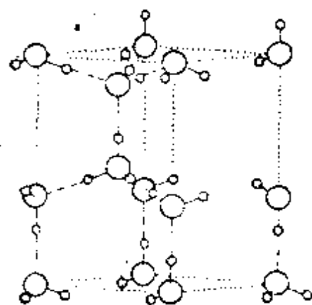
图 10.13 冰- \text{I}_h 的结构
