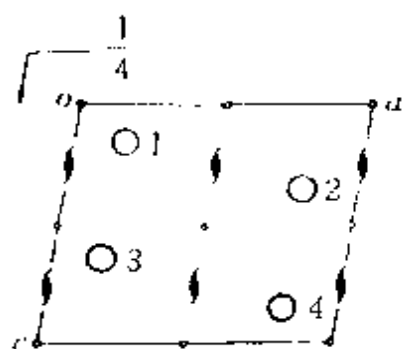
图 7.13 C_{2h}^5-P2_1/c 的等效点系
