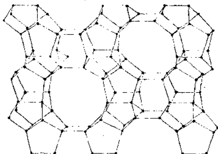
图 9.19 ZSM-5 型分子筛骨架的结构
