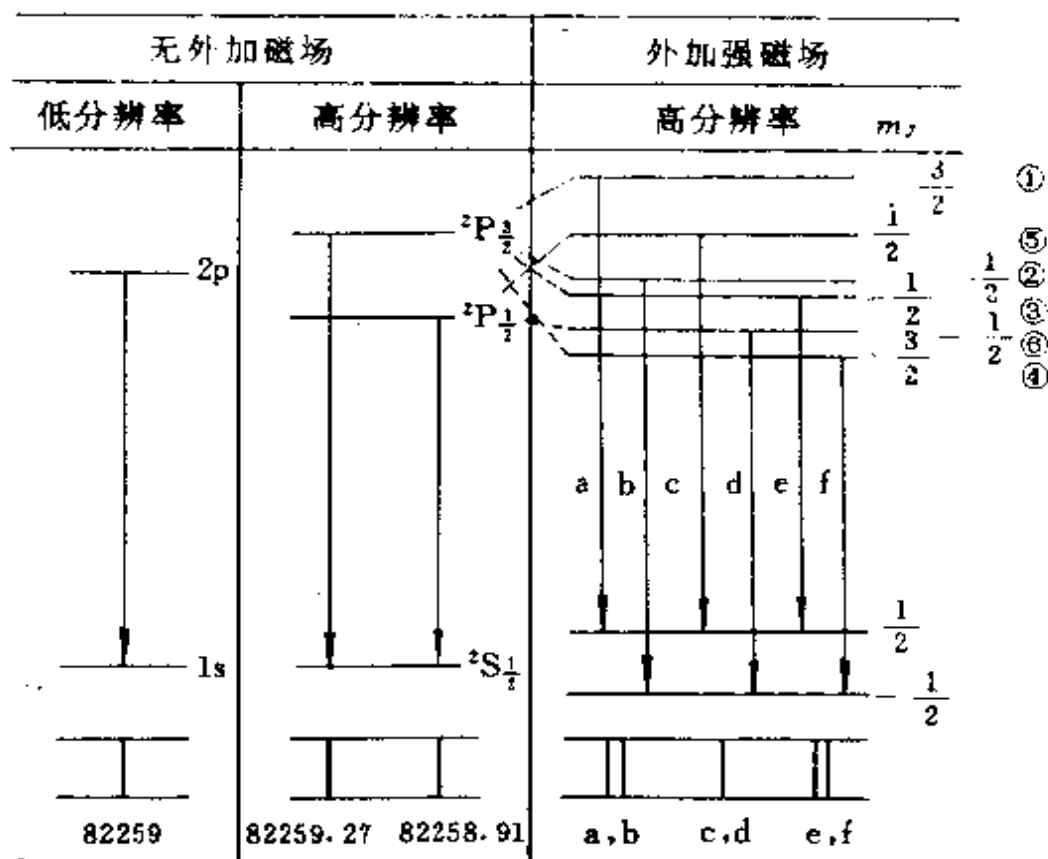
图 2.11 H 原子 2p \rightarrow 1s 跃迁的能级和谱线
