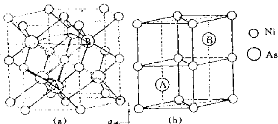
图 9.3 NiAs 的结构
