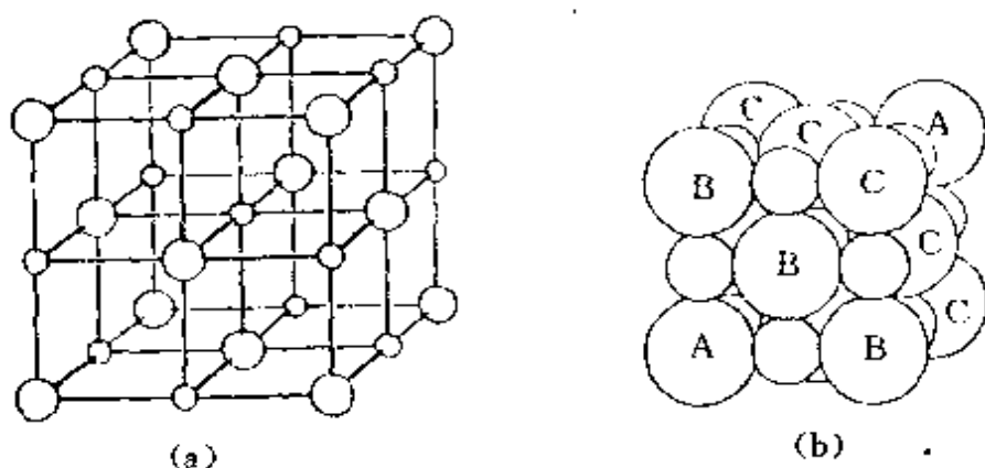
图 9.2 NaCl 的结构
