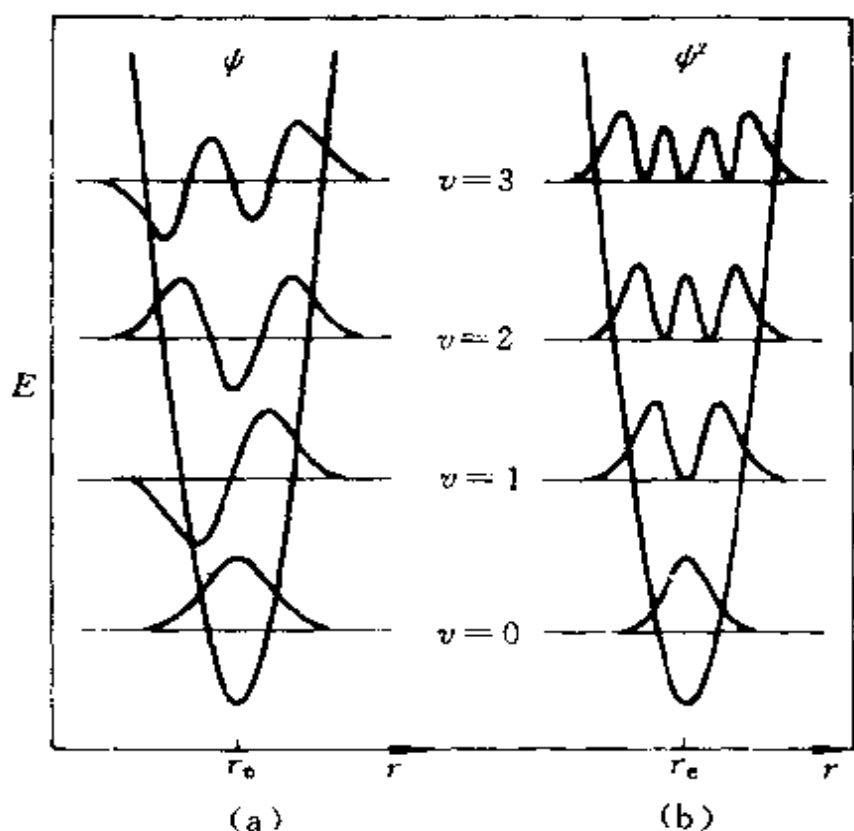
图 3.18 简谐振子的 \psi-r 图(a)和 \psi^2-r 图(b)
