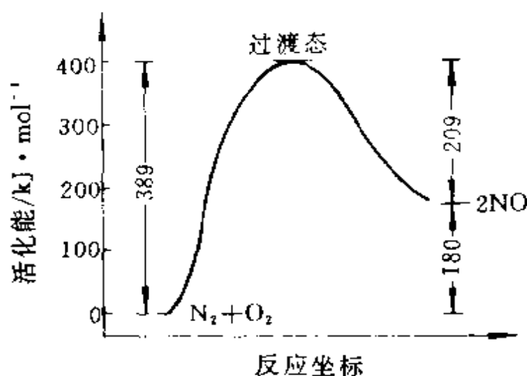
图 5.13 \text{N}_2 + \text{O}_2 \longrightarrow 2\text{NO} 的反应过程
